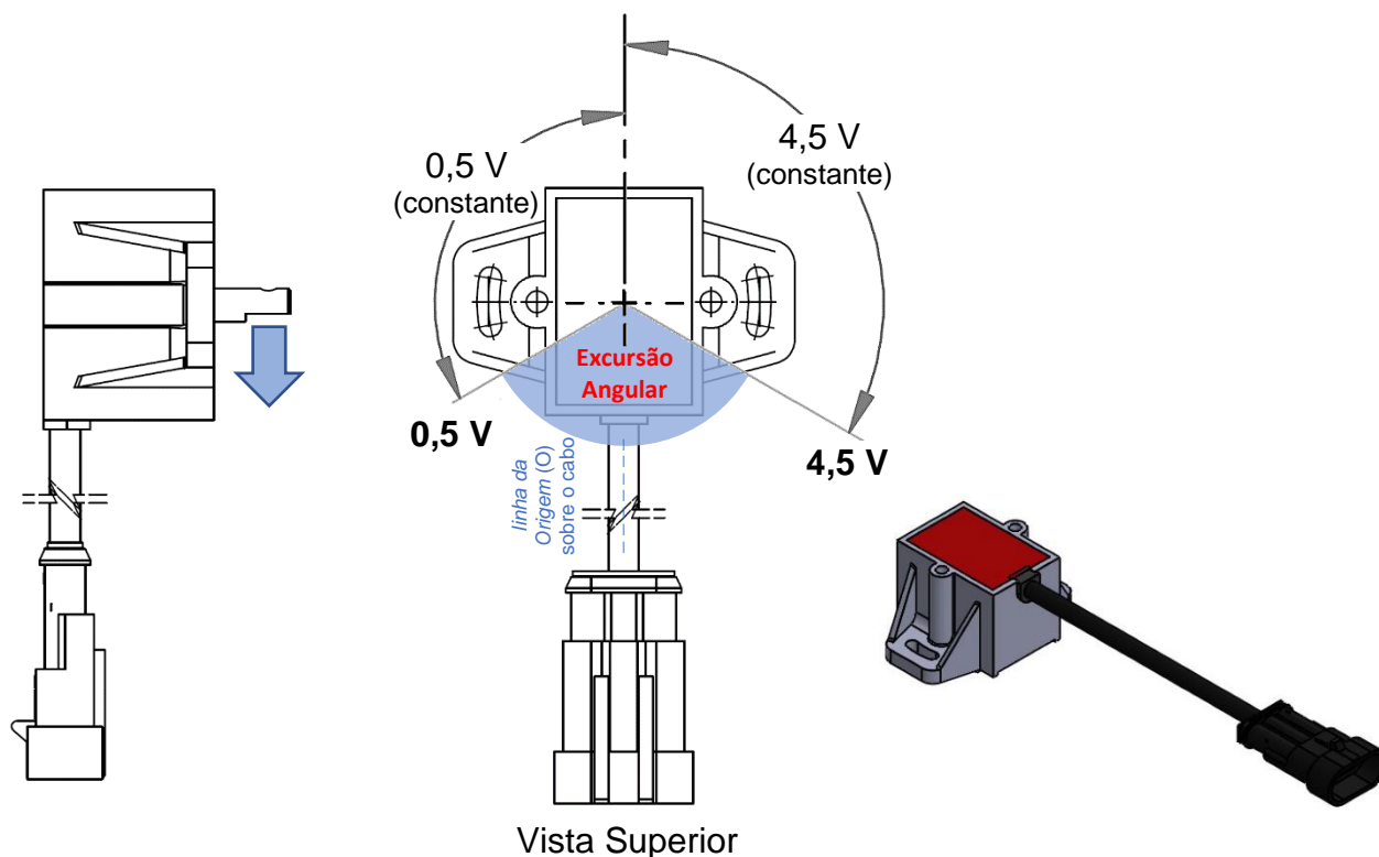
Figura 7 - Representação da Excursão Angular
