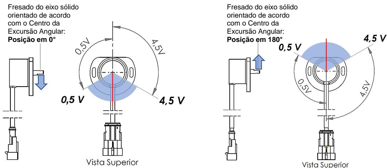
Figura 5 – Referenciamento do eixo sólido de acordo com o Centro da Excursão Angular
