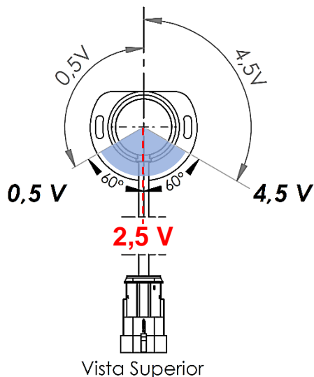
Figura 6 – Magnitude do sinal no Centro da Excursão Angular
