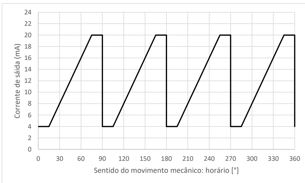
Figura 13 - Ângulo de excursão 60°, módulo 4 (4 curvas), Centro da Excursão Angular em 45°, 135°, 225°, e 315°, sentido de incremento horário, 4-20 mA
