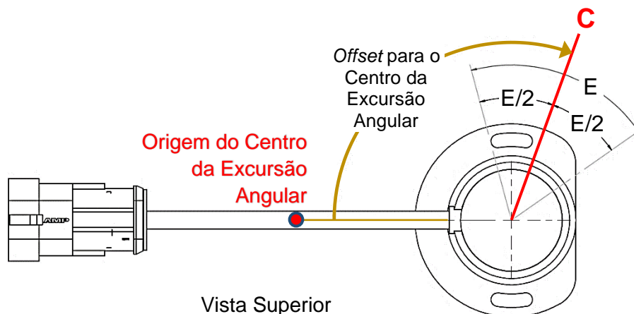
Figura 4 - Representação do Centro (C) da Excursão Angular (E)
