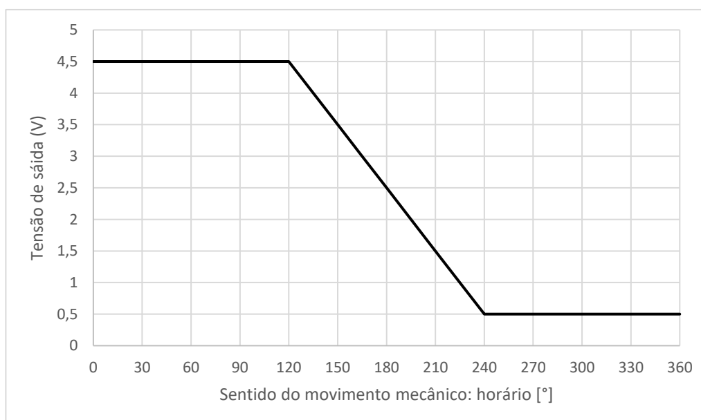
Figura 11 - Ângulo de Excursão 120°, Centro da Excursão Angular em 180°, sentido de incremento anti -horário (0,5-4,5 V)
