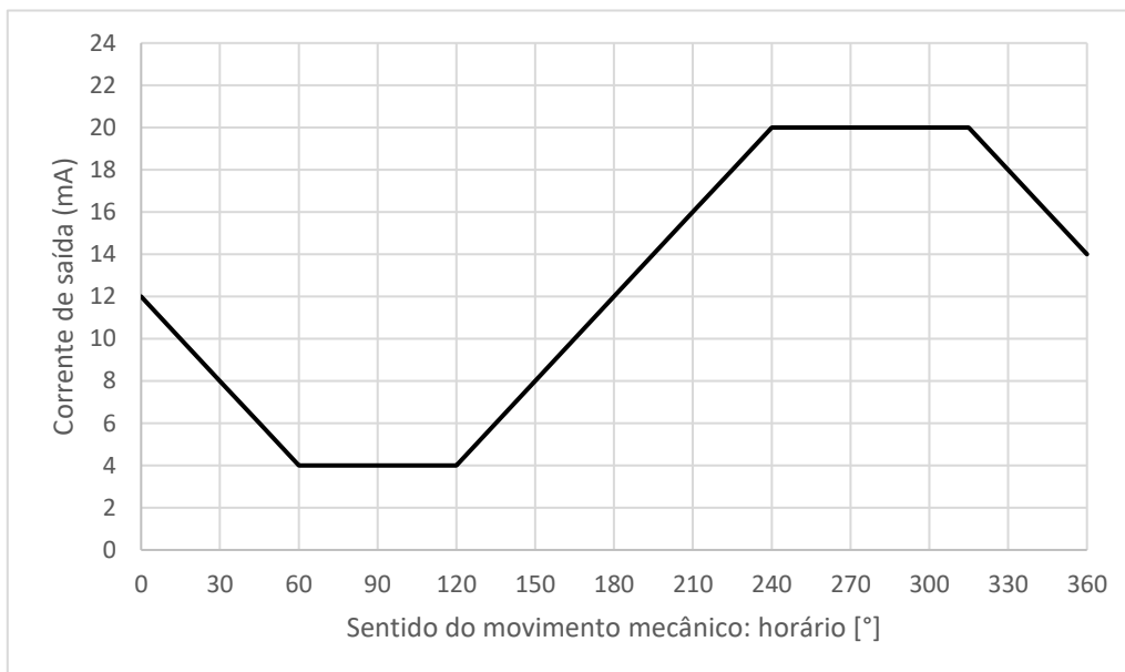
Figura 12 - Ângulo de Excursão 120°, Centro da Excursão Angular em 0°, sentido de incremento anti -horário (e Centro da Excursão Angular em 180°, sentido de incremento horário), curva-dupla espelhada (trapezoidal), 4-20 mA
