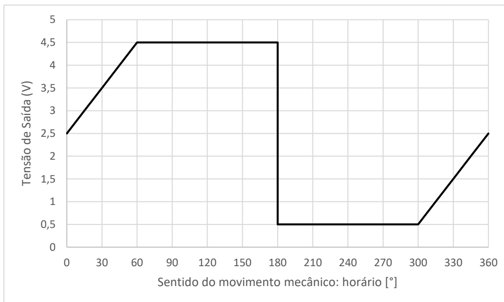
Figura 10 - Ângulo de Excursão 120°, Centro da Excursão Angular em 0°, sentido de incremento horário (0,5-4,5 V)
